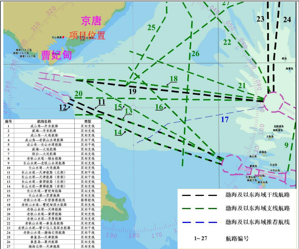
图4.2-1 本项目附近水域习惯航路分布图
