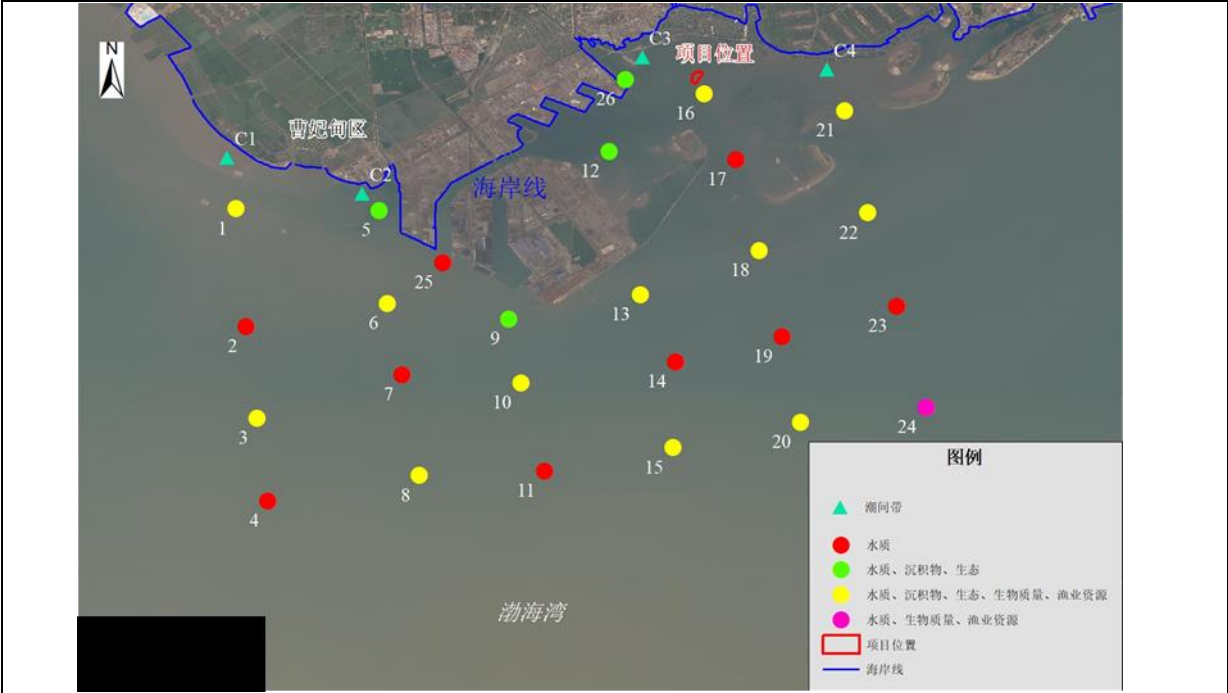
图2.2-14 海域环境质量现状调查站位图
